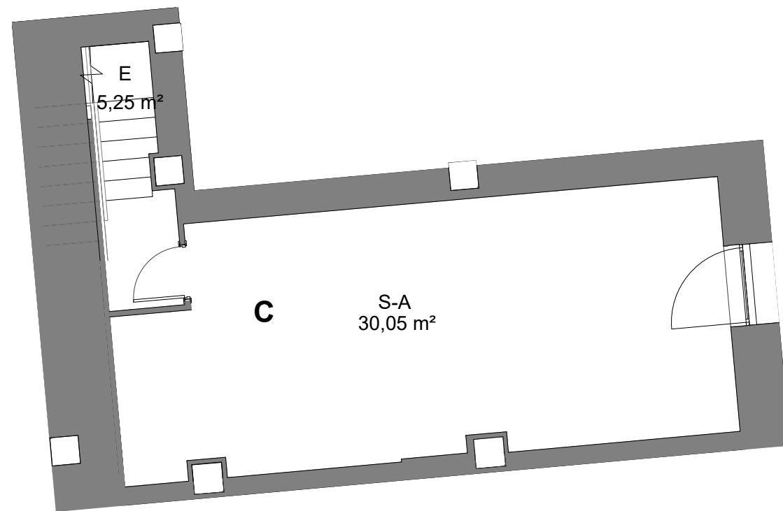
PLANTA SÓTANO
