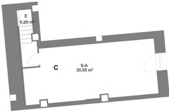
PLANTA SÓTANO (ESTADO ACTUAL)
